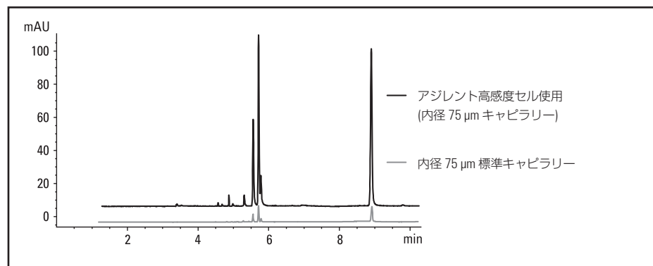
ナフタレンスルホン酸の分析におけるアジレント高感度セルと内径 75 \mu m 標準キャピラリーの比較
