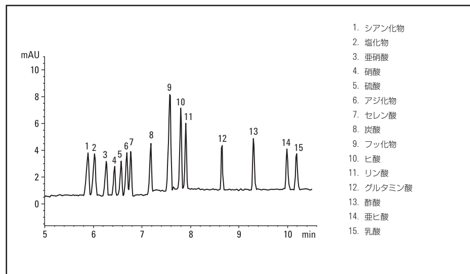
有害陰イオン分析キットでの陰イオン標準液の分析
