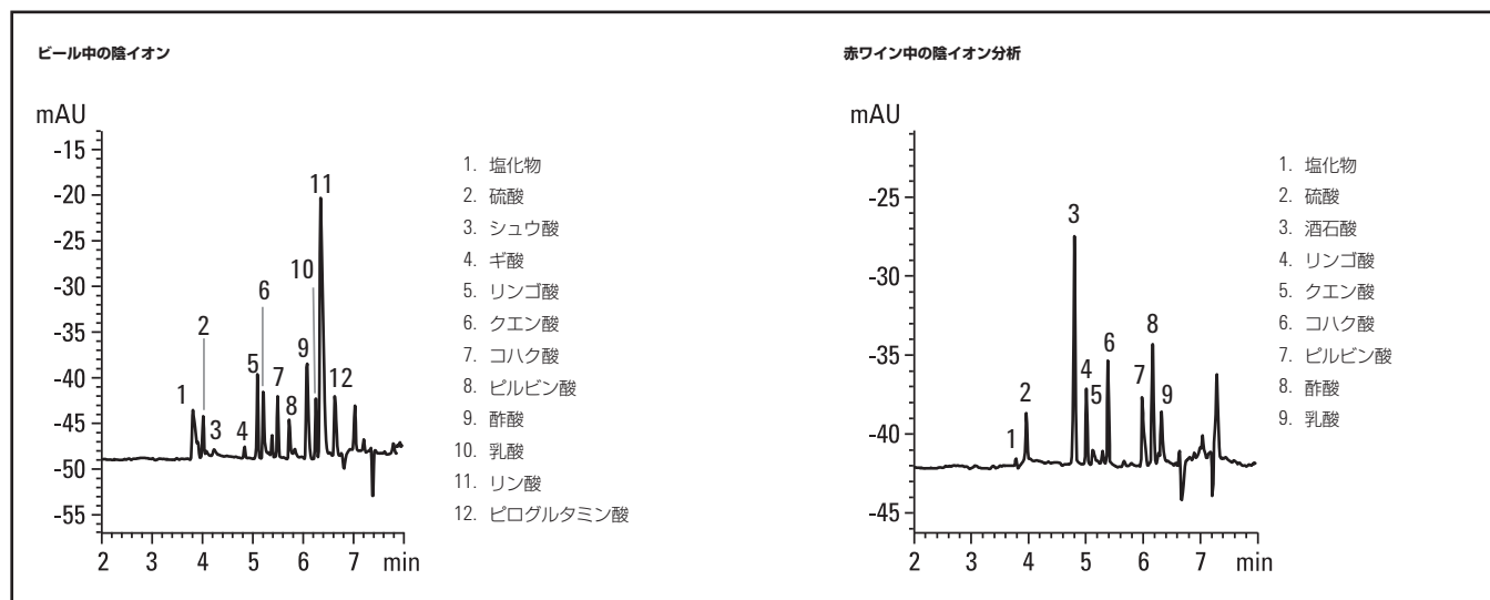
ビールおよび赤ワイン中の有機酸
