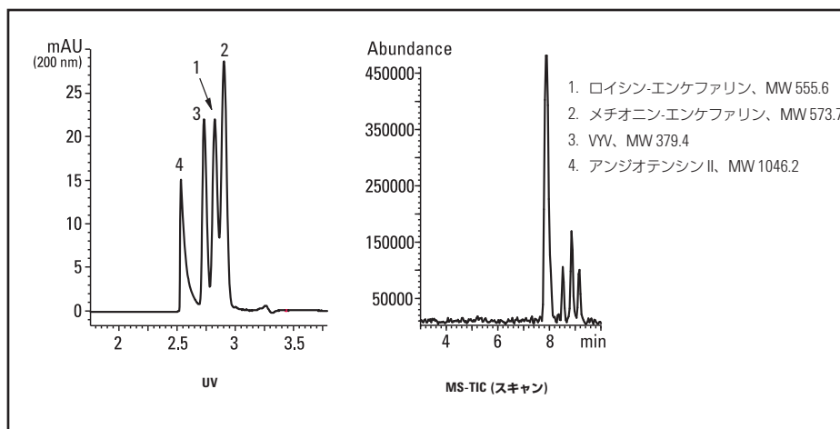
4 成分ペプチド混合物 (210 fmol) の CE/MS 分析
