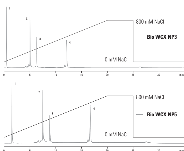
Agilent Bio WCX NP5 と Agilent Bio WCX NP3 によるタンパク質分離
