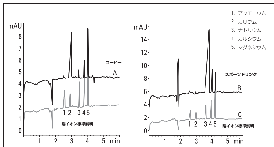
コーヒーとスポーツドリンク中の陽イオン分析
