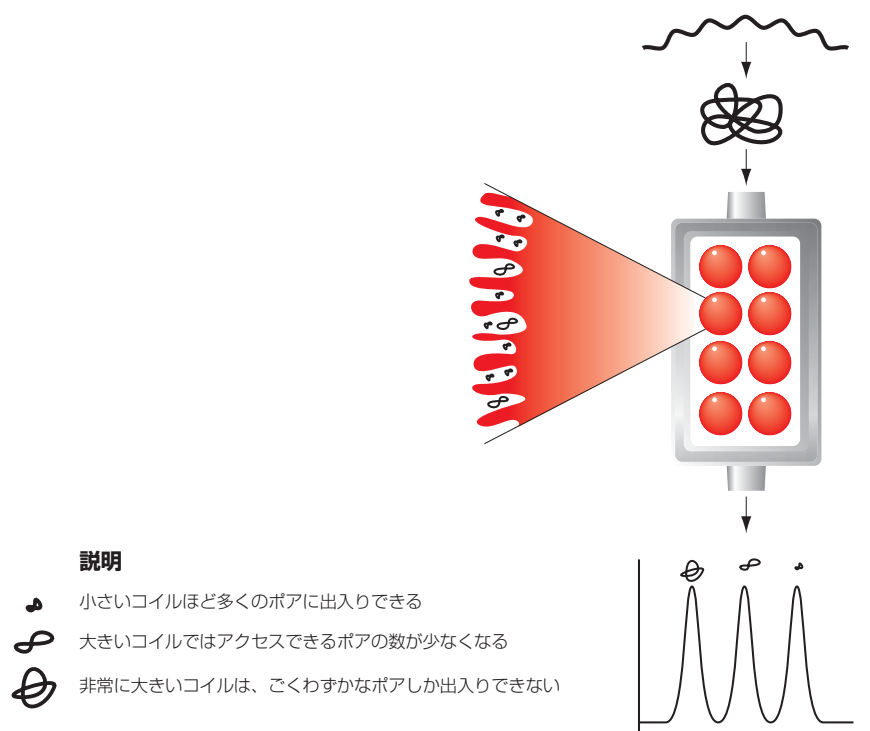
GPC と SEC のメカニズム
