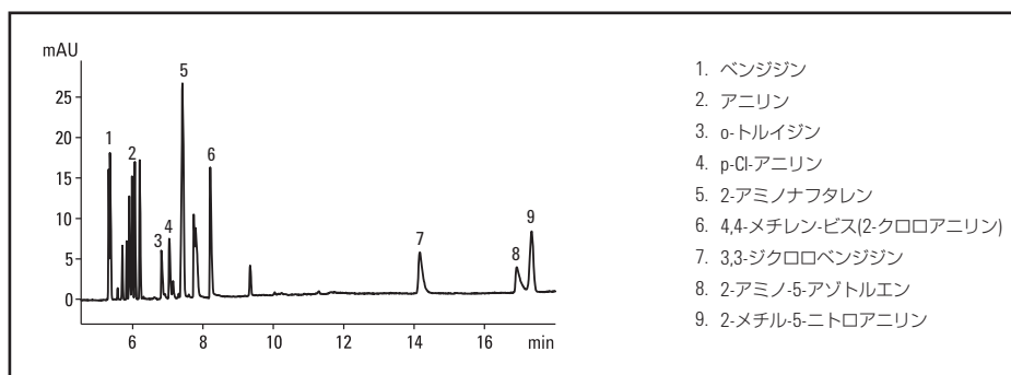
PVA コーティングキャピラリーを使った塩基性アミン (アゾ染料の分解生成物) の CZE 分析
