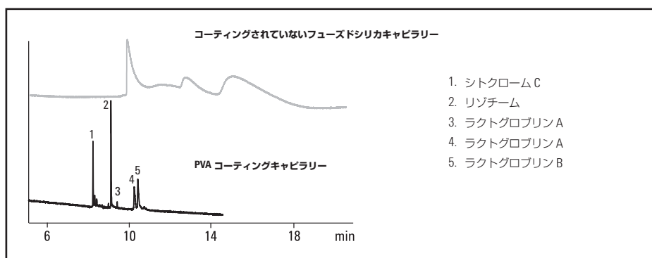
タンパク質の吸着を抑制する PVA コーティングキャピラリー
