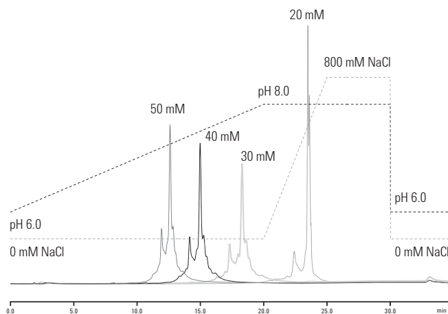
異なる条件における IgG モノクローナル抗体の分離
