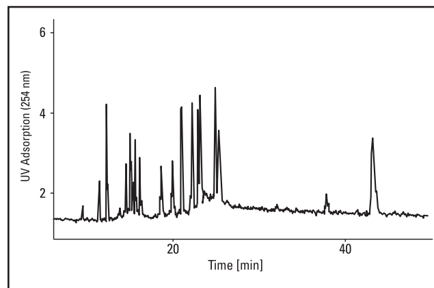
\mu SIL-WAX を用いたミオグロビントリプシン消化物の分析
