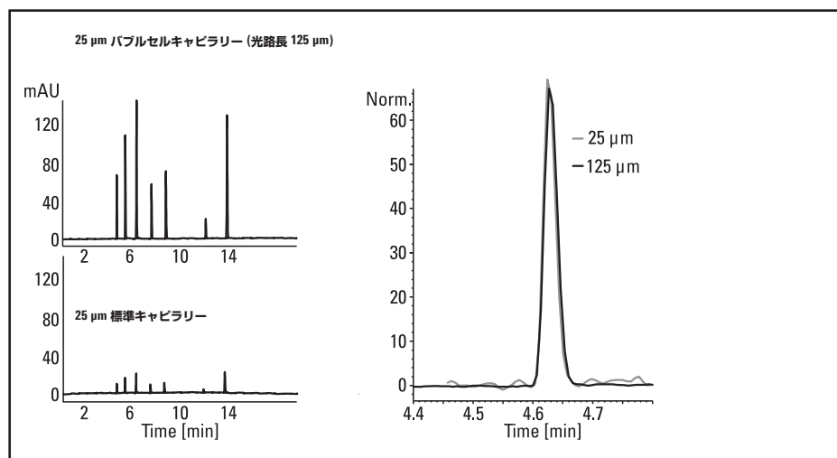
内径 25 \mu\text{m} 標準キャピラリーとバブルセルキャピラリーを用いた風邪薬原料の分析
