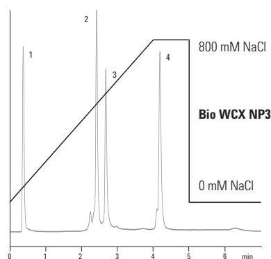
Agilent Bio WCX NP3 と Agilent Bio WCX NP1.7 の比較 (流量 1.0 mL/min)
