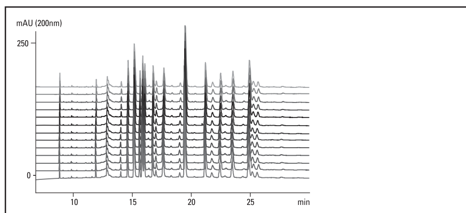
内径 75 \mu\text{m} の標準フューズドシリカキャピラリーを用いた、組み換えヒト成長ホルモンのトリプシン消化物の CZE
