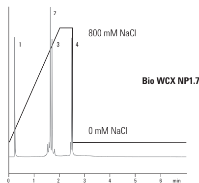
Agilent Bio WCX NP1.7 による 3 分未満でのタン パク質の分離 (流量 1.7 mL/min)。
