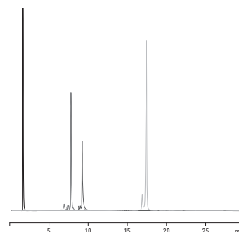
Agilent Bio WCX、NP5 カラムを使用した pH 6.5 におけるタンパク質標準の分離
