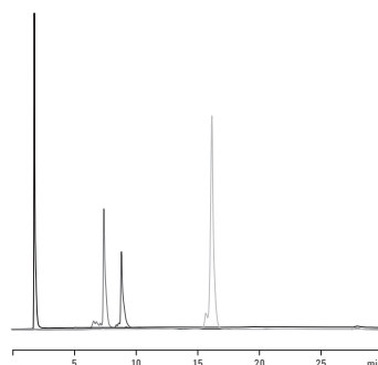
Agilent Bio WCX、NP10 カラムを使用した pH 6.5 におけるタンパク質標準の分離
