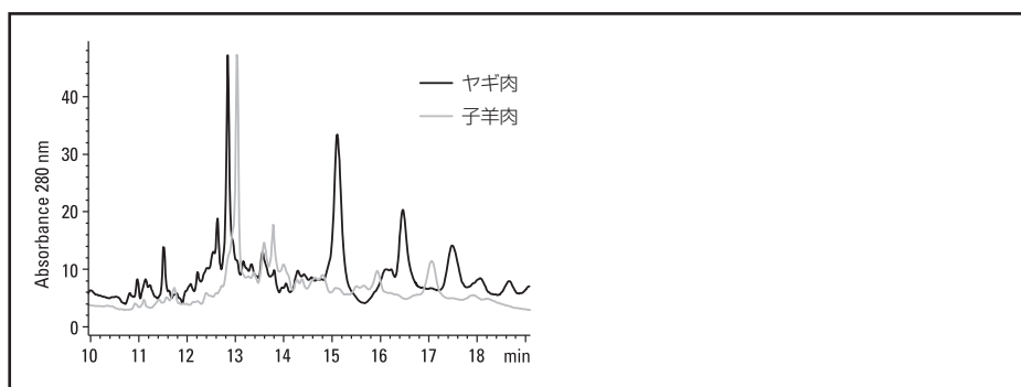
PVA コーティングキャピラリーを使用した食肉タンパク質の等電点電気泳動
